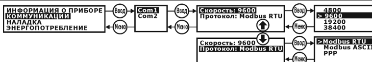
Рис. 3.10 – Настройка Com-портов
