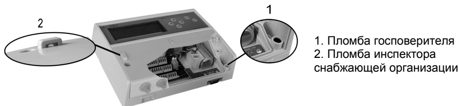
Рис. 1.2 – Места пломбирования вычислителя
